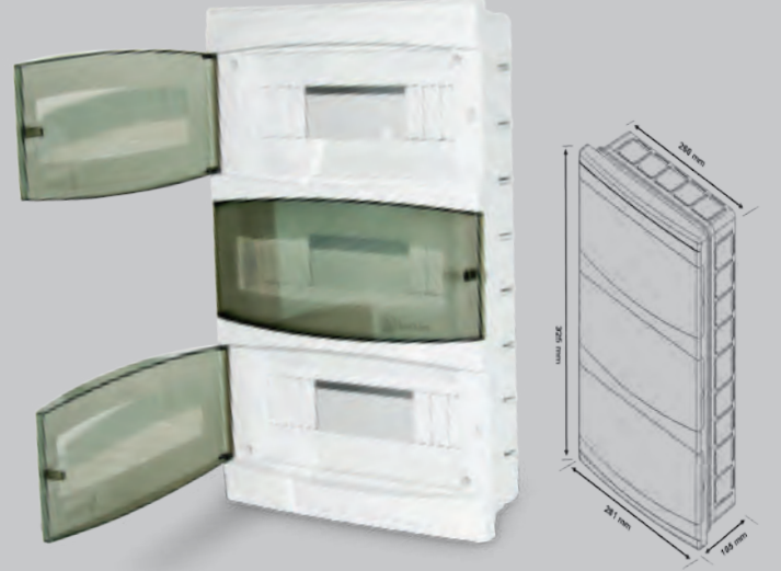
36'lü Sıva Altı Sigorta Kutusu 36 Module Distribution Box - Recessed
